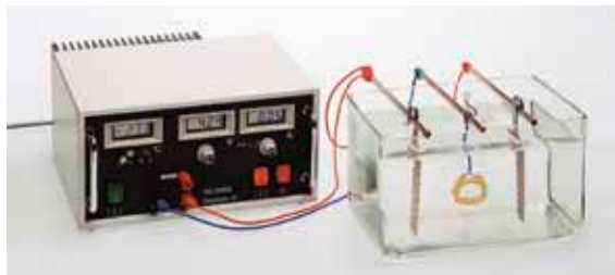
Kleinanlage für Goldschmiede für den galvanischen Überzug von Schmuck. BILD: UBOS
